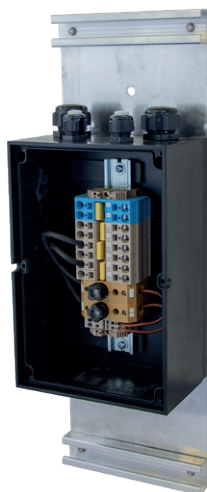
Mastverteiler 58 Typ 300
